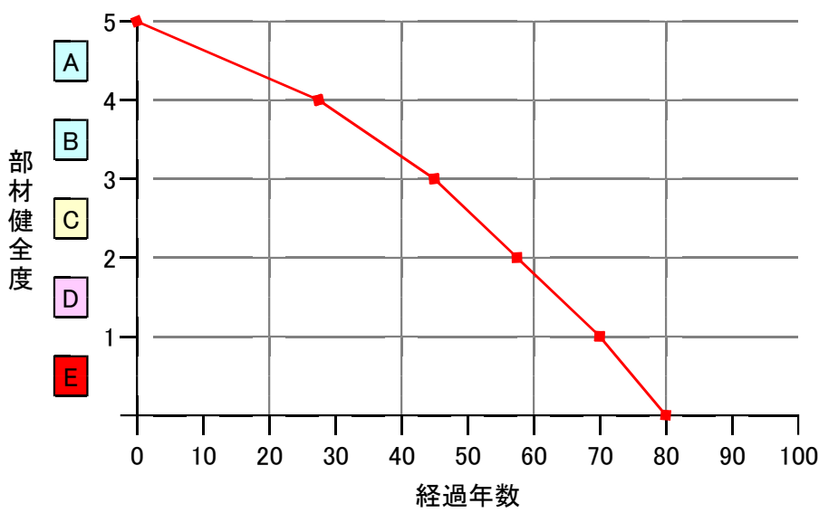
d) コンクリート橋:コンクリート床版
