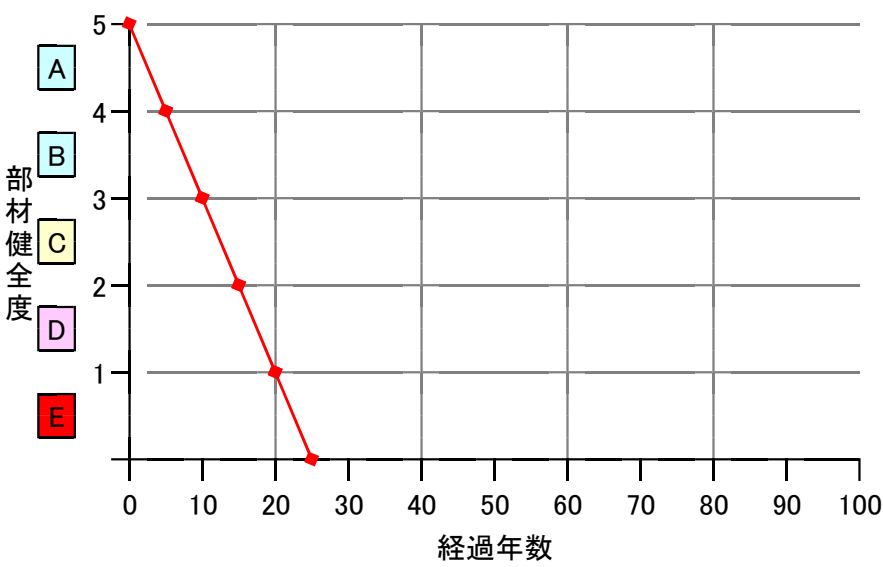
g) 伸縮装置(ゴムジョイント)
