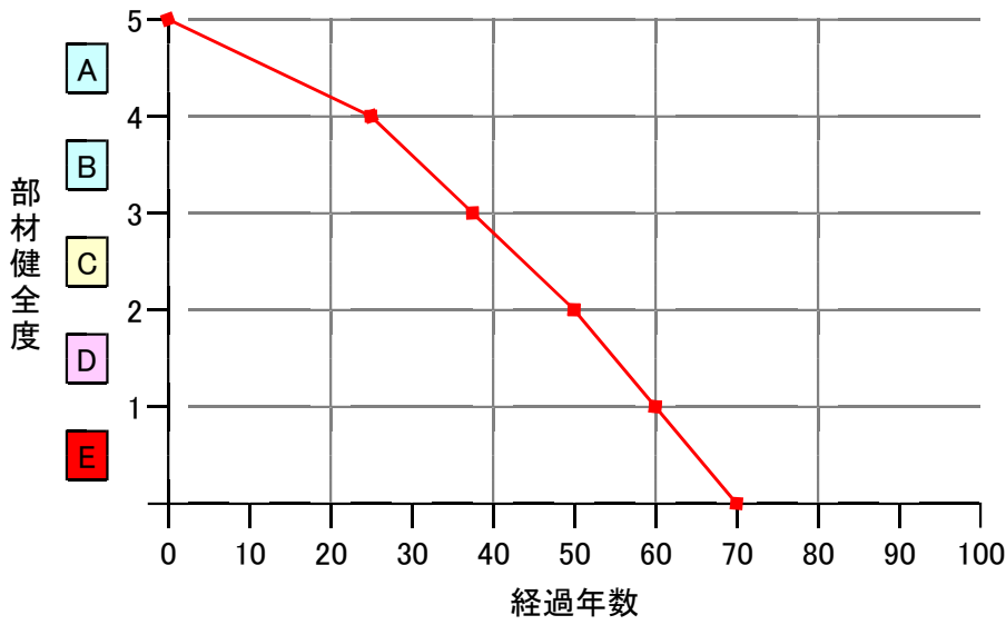
b) 鋼橋:コンクリート床版
