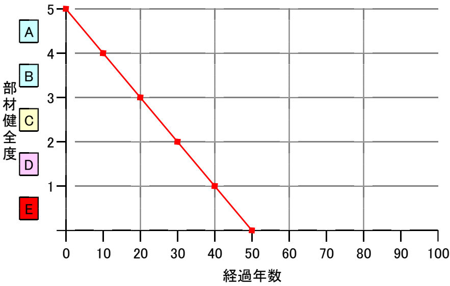
a) 鋼橋:主構(普通鋼材+普通塗装)
