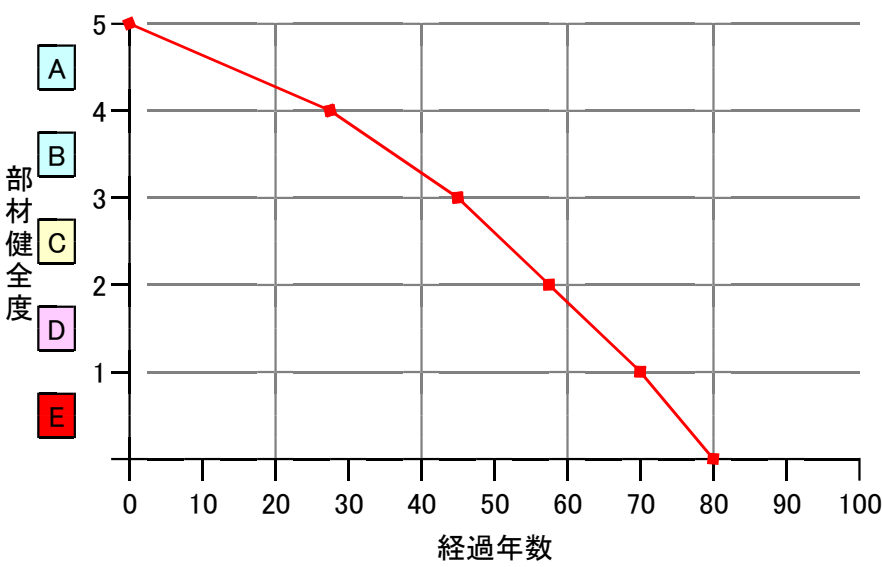
c) コンクリート橋:主構
