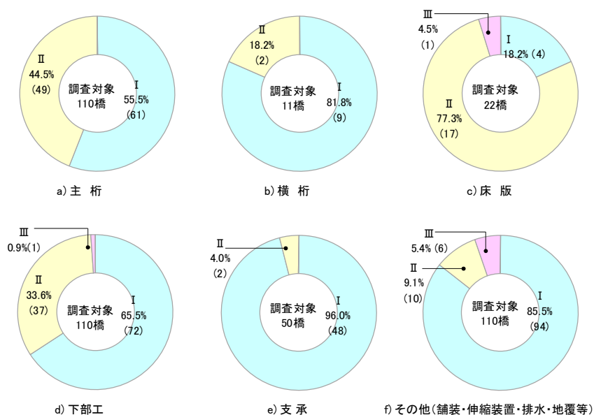
図-3 定期点検結果の健全性評価の割合 (部材別)
