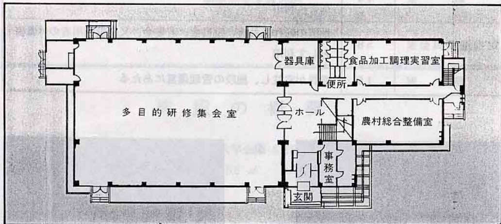
1F 平 面 図
