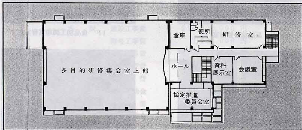
2F 平 面 図
